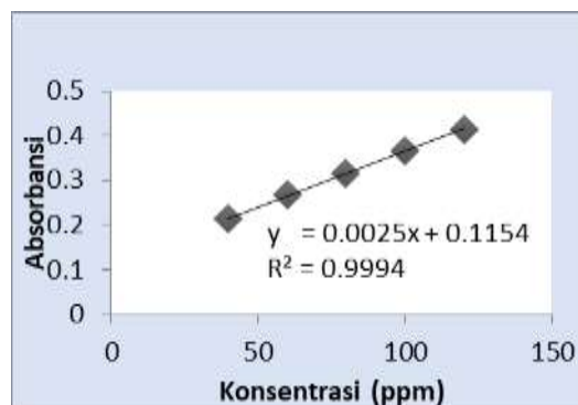
Gambar 2 Regresi Linier Asam Kojat dalam Dapar Phosphat
