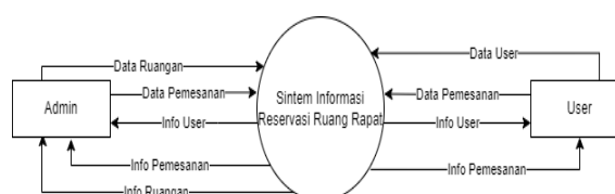
Gambar 2. Diagram Konteks
