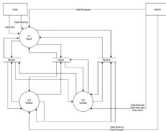
Gambar 4. DFD Level 2
