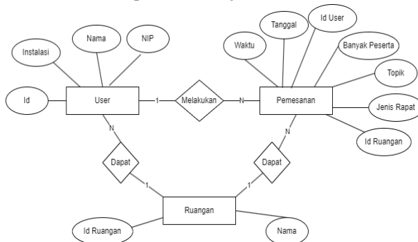
Gambar 7. ERD
